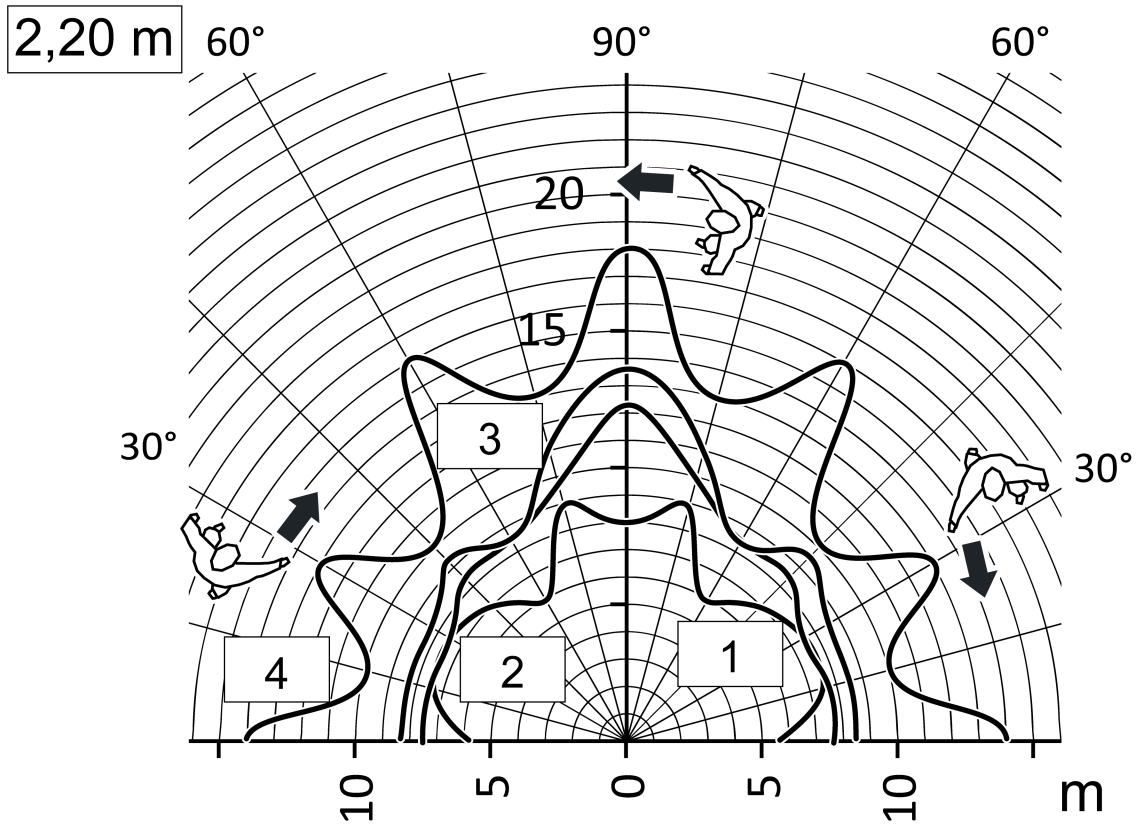
Рисунок 9: Дальность действия при направлении движения по касательной, монтажная высота 2,20 м
