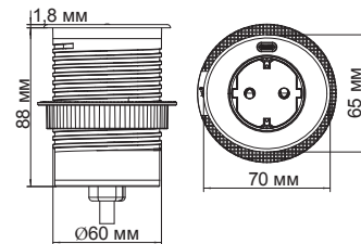
Рис. 1. Габаритные размеры
