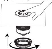
Рис. 2. Схема монтажа
