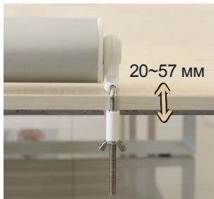
Рис. 2. Пример монтажа
