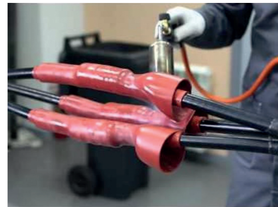
Подключение и защита любых типов кабеля до 35 кВ
